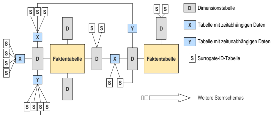
Abbildung 1: SAP Sternschemas
